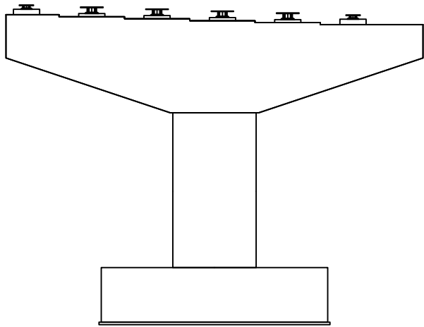
정 면
