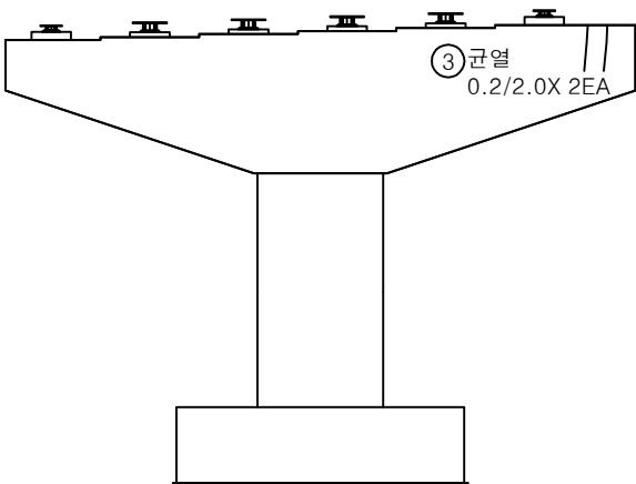
배 면
