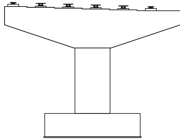
정 면
