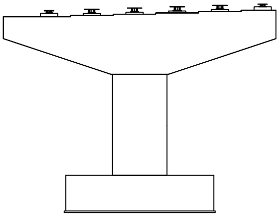
배 면
